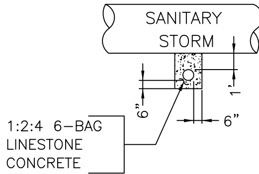
A-A
